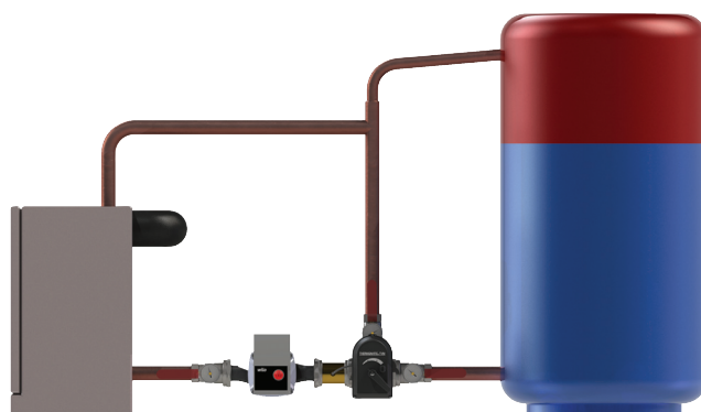
Пример установки Thermomatic TVM для контроля температуры возвратной воды в котел, Laddomatic.
